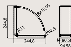
KÖNYÖK CRO 90 220X90 MM FUN 112.0459.455
