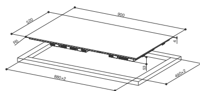
HAGYOMÁNYOS (STANDARD) BEÉPÍTÉS
