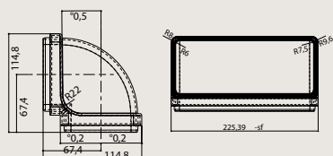
KÖNYÖK CRV 90 220X90 MM FUN 112.0459.453
