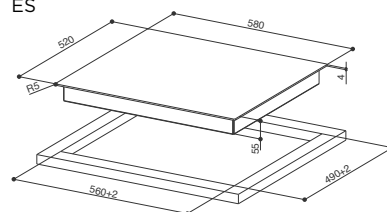
HAGYOMÁNYOS (STANDARD) BEÉPÍTÉS
