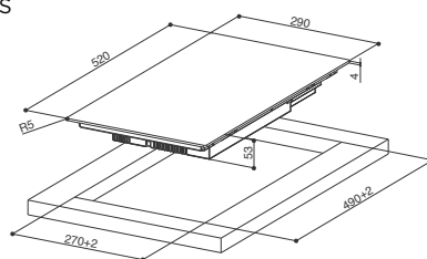
HAGYOMÁNYOS (STANDARD) BEÉPÍTÉS
