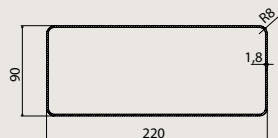
NÉGYSZÖGLETES CSŐ TR 1200 220X90 MM FUN 112.0459.427
