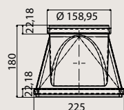
CSATLAKOZÓ RRC 220X90 MM FUN 112.0459.429
