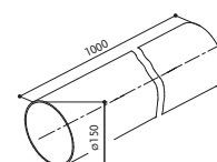
LÉGTECHNIKAI TC 1000 Ø 150 MM FUN 112.0253.681
