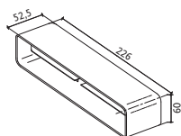
NÉGYSZÖGLETES CSATLAKOZÓ FUN 112.0157.295
