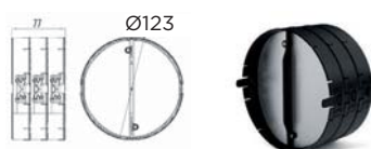
LÉGELZÁRÓ SZELEP 3D D125 FUN 112.0569.782
