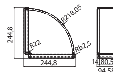
LÉGTECHNIKAI TC 1000 Ø 150 MM FUN 112.0253.681
