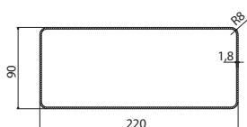
LAPOS CSATORNA TR 1200 220X90 MM FUN 112.0459.427
