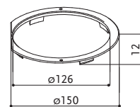
CSŐ - LAPOS CSATORNA ÁTALAKÍTÓ IDOM 2 FR FUN 112.0157.309
