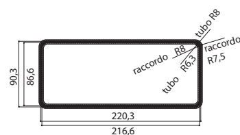
LAPOS CSATORNA CSATLAKOZÓ IDOM RCR 220X90 MM FUN 112.0459.428
