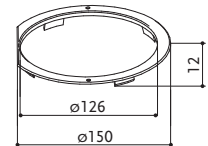
CSŐ - LAPOS CSATORNA ÁTALAKÍTÓ IDOM 2 FR FUN 112.0157.309
