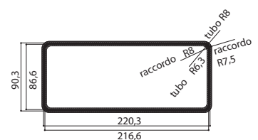
LAPOS CSATORNA CSATLAKOZÓ IDOM RCR 220X90 MM FUN 112.0459.428
